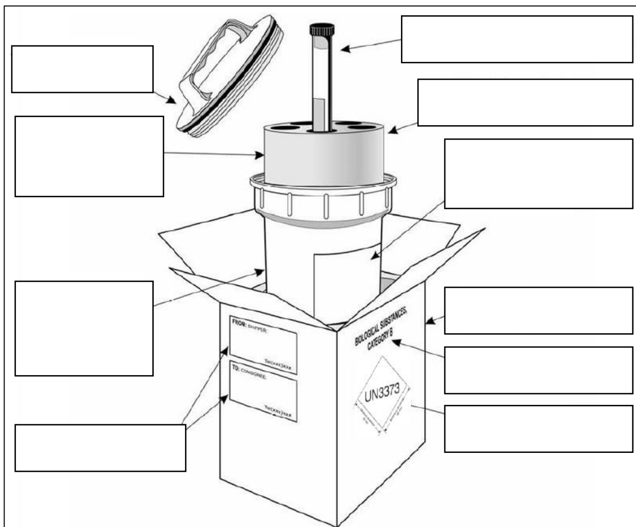
Diagrama 1: P650 Embalagens para substâncias biológicas, Categoria B (Imagem retirada de: Guia de orientação sobre regulamentos para o transporte de substâncias infecciosas 2015-2016. Organização Mundial de Saúde. Figura 9, Página 16)
